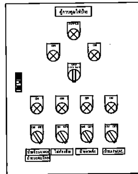
ด้านหน้า
